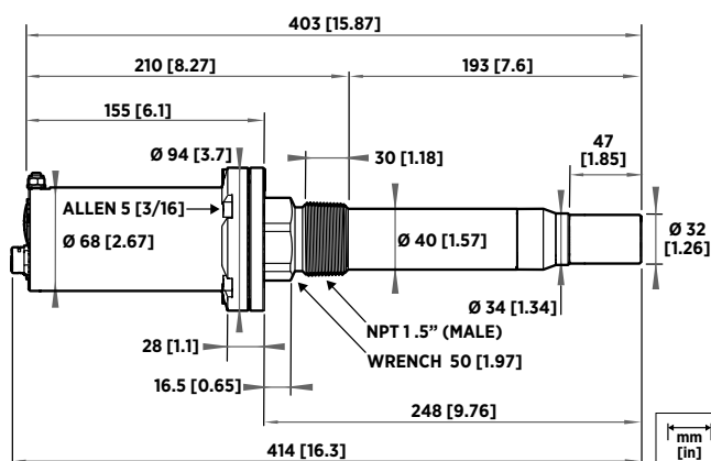
MGP262 dimensions
