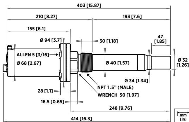
MGP261 dimensions
